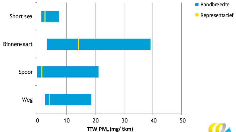
Figuur 4 Overzicht emissiefactoren fijnstof (PM v ) - containers (tank -to-wheel) (g/tkm)
