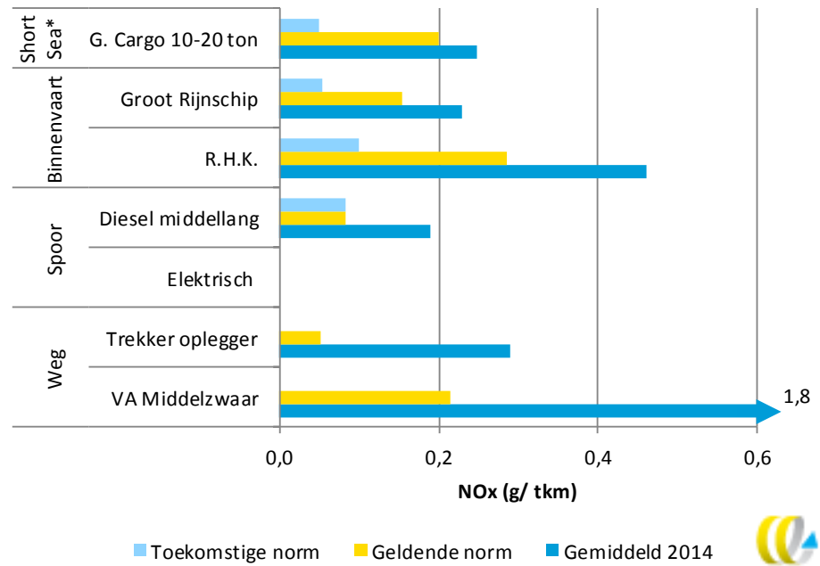
Figuur 8 TTW NO x -emissies gemiddeld 2014, emissies voor bulk transport. Gemiddeld 2014, geldende norm 2014 en toekomstige norm vergeleken
