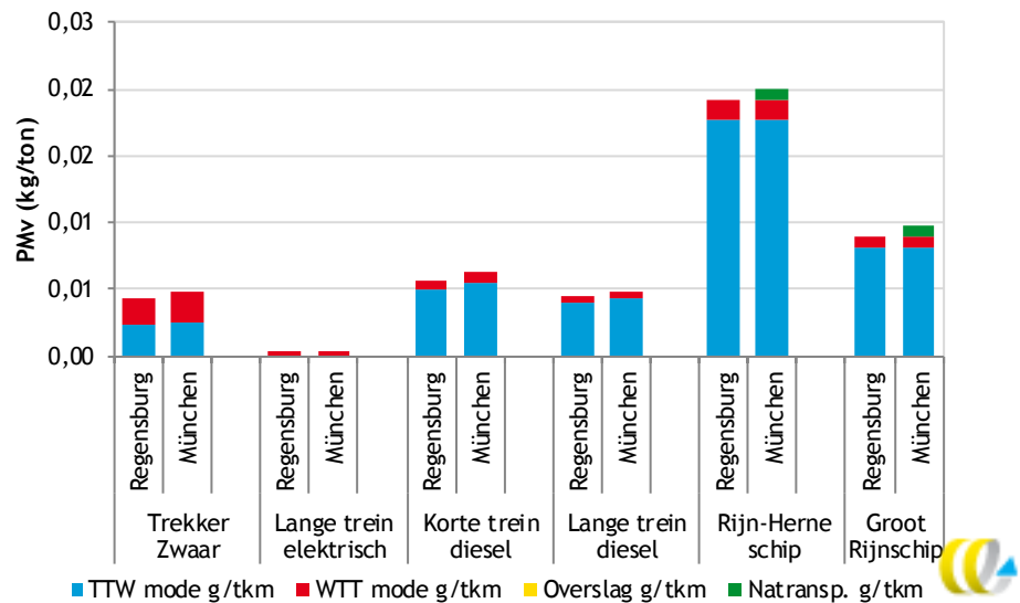
Figuur 17 PM v -emissies per tkm voor zwaar bulktransport; case: Amsterdam-Regensburg
