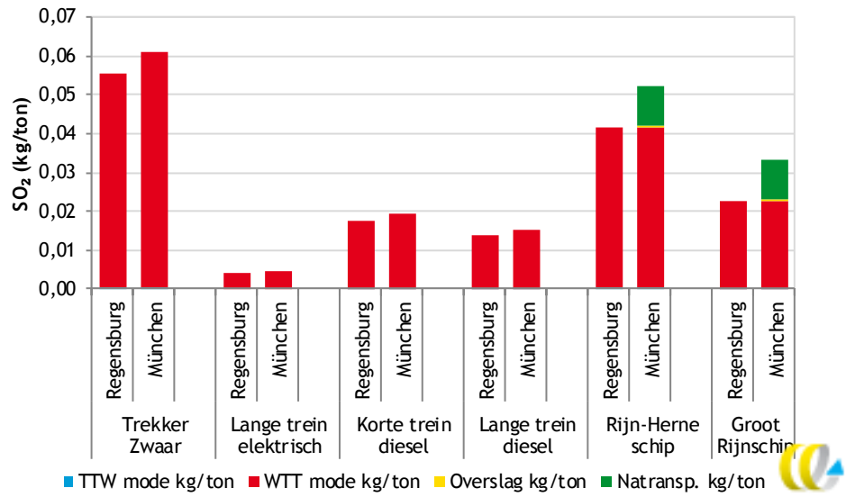
Figuur 16 SO 2 -emissies per tkm voor zwaar bulktransport; case: Amsterdam-Regensburg
