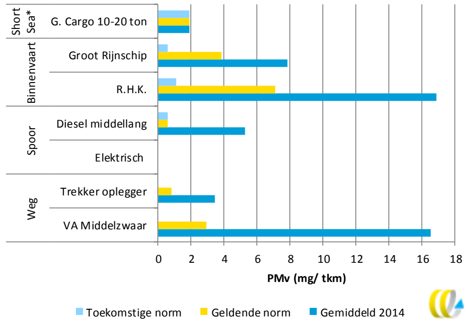
Figuur 7 TTW fijnstof (PM v )-emissies voor bulk transport. Gemiddeld 2014, geldende norm 2014 en toekomstige norm vergeleken
