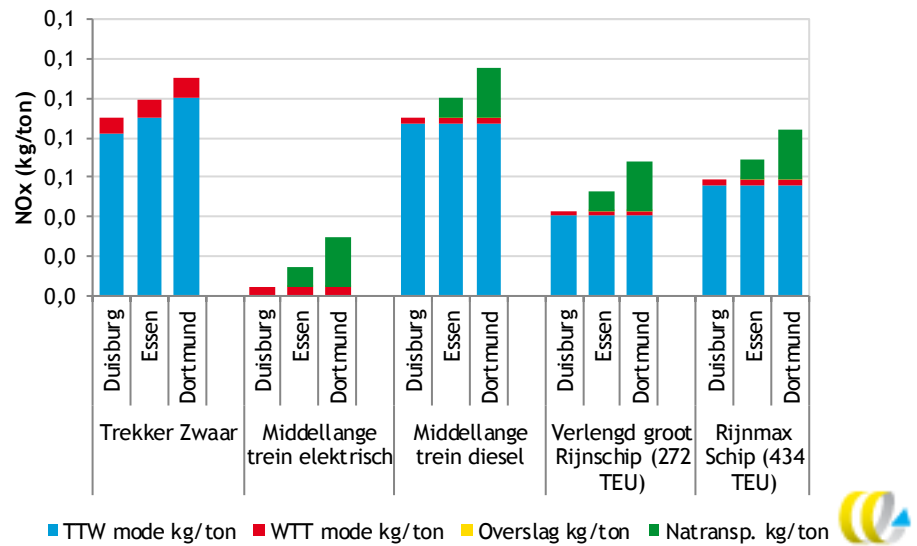
Figuur 14 NO x -emissies per ton voor middelzwaar containertransport; case: Rotterdam-Duisburg
