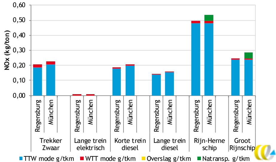
Figuur 18 NO x -emissies per tkm voor zware bulktransport; case: Amsterdam-Regensburg
