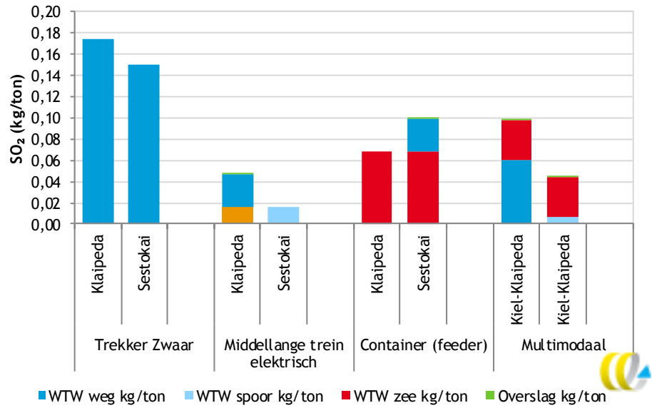
Figuur 20 SO 2 -emissies per ton voor middelzwaar containertransport; case: Rotterdam-Litouwen
