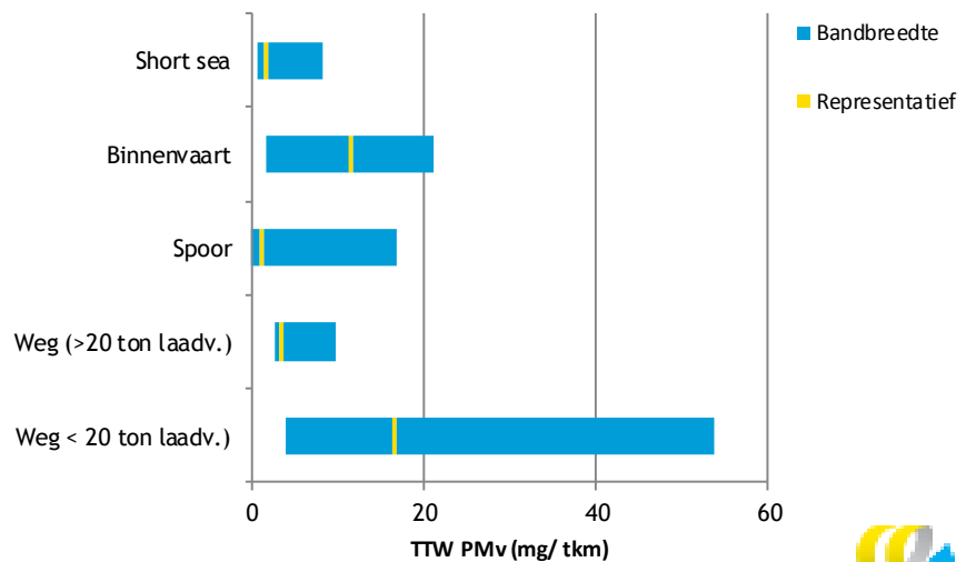
Figuur 3 Overzicht emissiefactoren fijnstof (PM v ) - bulk/stuks (tank -to-wheel) (g/tkm)
